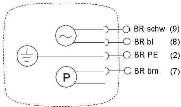
Connexion au contrôle de la pompe / Base de contrôle dans la boîte de jonction.
